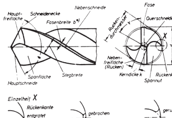
Aresta principal · Face de saída · Aresta transversal · Guia · Canal
