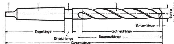
Haste cônica · Lingueta de extração · Canal · Ponta · Diâmetro da broca
